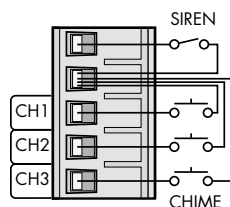
10) Anschluss Gongtaster/SirenenSchalter
